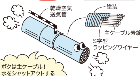
ケーブル表面拡大図
